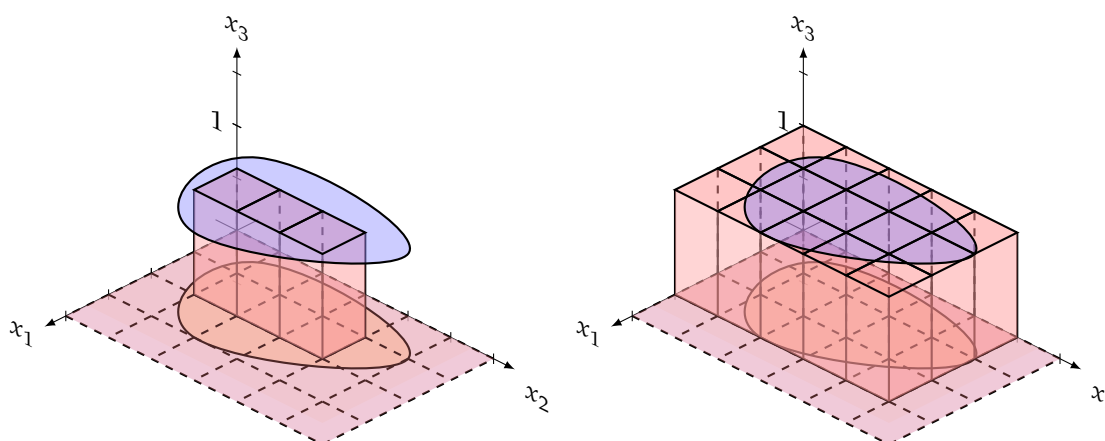
Abbildung 4.3: Unter- und Obersumme bezüglich \mathbb{1}_J zu einer bestimmten Zerlegung
